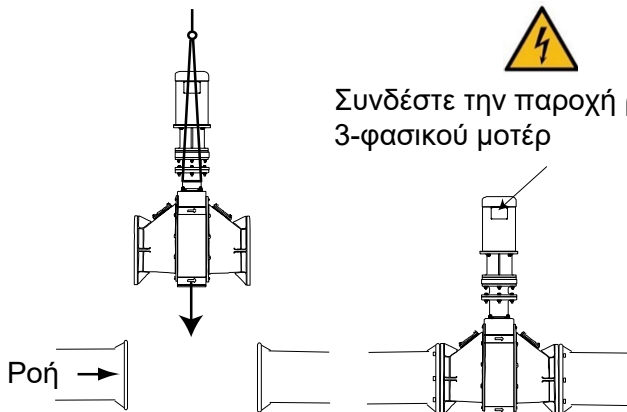
Εγκατάσταση εντός γραμμής
