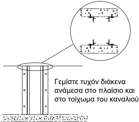
Πλαίσιο (μέσα στο κανάλι)
